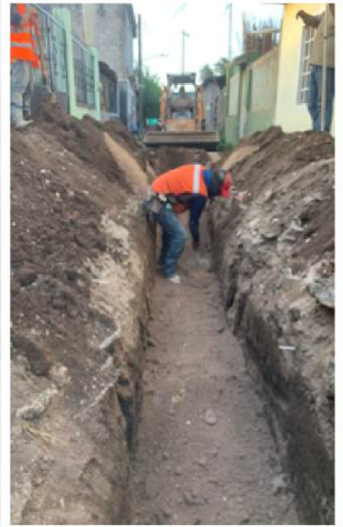
Construcción de drenaje sanitario en el sector oriente de Rioverde (ZAP 046A) en calles Verástegui, San Francisco de Asís y Noche Buena.
