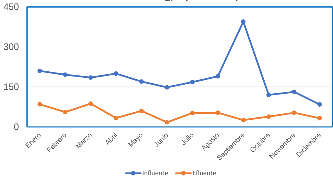
Comportamiento anual de Solidos Suspendidos Totales en mg/L (año 2018)
