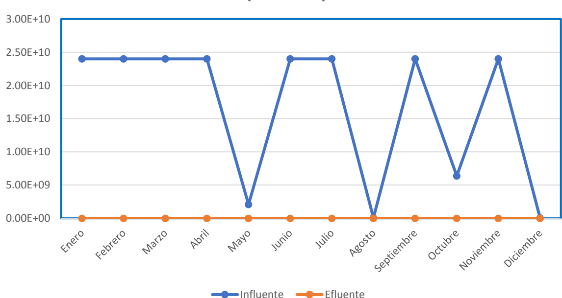
Comportamiento anual de coliformes fecales NMP/100 mL (año 2018)
